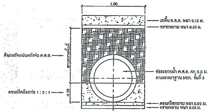
รูปตั้งที่ปลายท่อแบบแถวเดี่ยว มาตราส่วน 1:20
