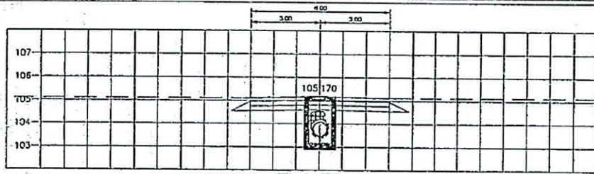
STA. 0+275.000 NGL = 105.170
