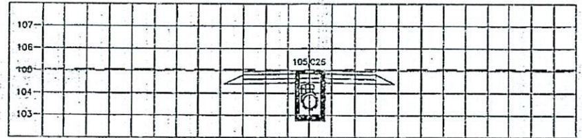
STA. 0+350.000 NGL = 105.025
