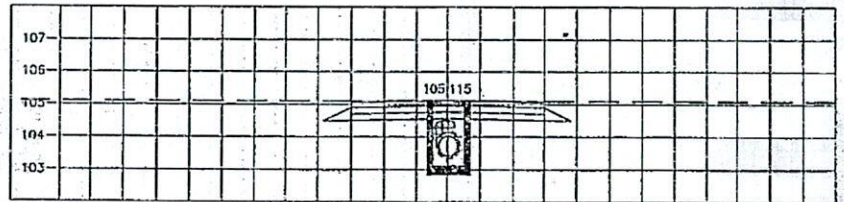
STA. 0+325.000 NGL = 105.115
