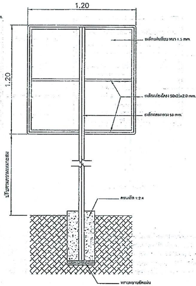
รูปด้านหลัง 1:15
