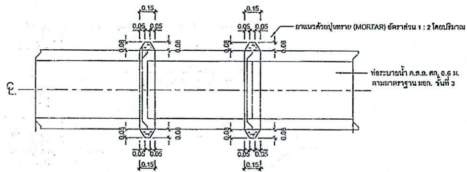
รูปตัดแสดงการต่อท่อยาแนว มาตราส่วน 1:20
