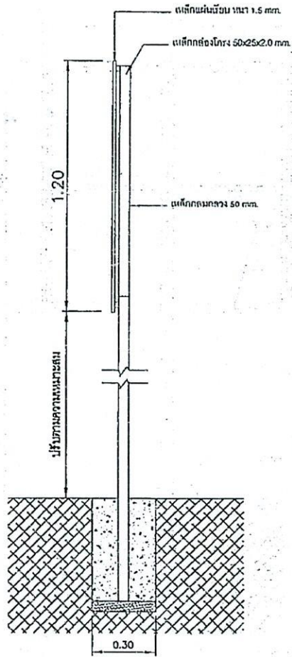
รูปด้านข้าง 1:15
