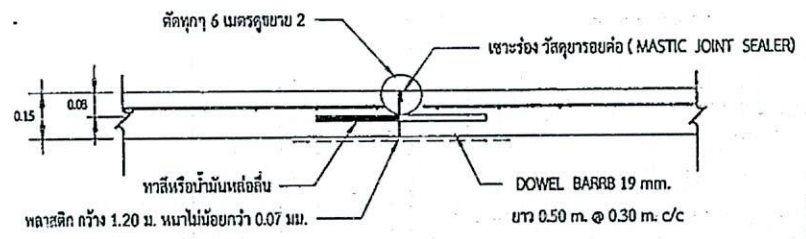
ขยายรอยต่อเพื่อการก่อสร้าง CONSTRUCTION JOINT
