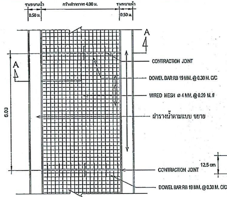
แปลนแสดงการเสริมเหล็กและรอยต่อ
