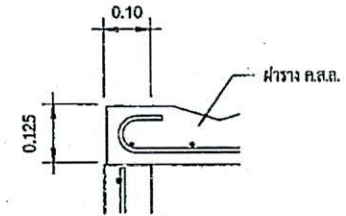
ขยายขอบระบายน้ำ มาตราส่วน 1:10
