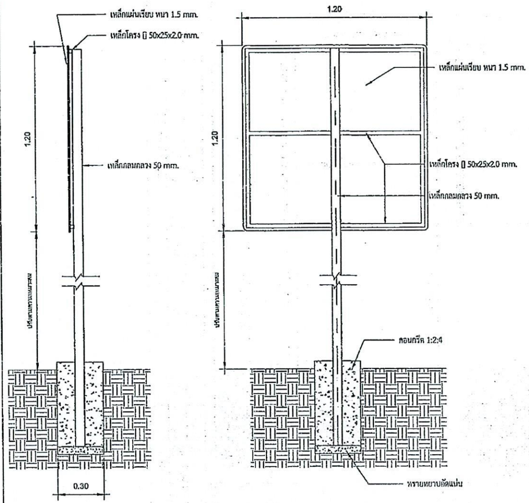
รูปด้านข้าง 1:15
