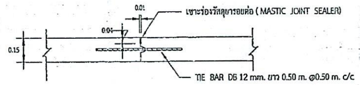
ขยายรอยต่อ LONGITUDINAL JOINT
