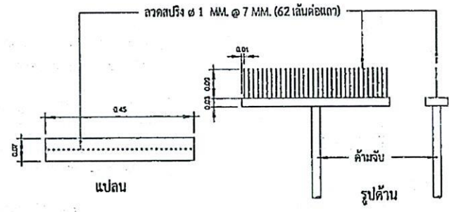
แบบขยายไม้กวาดผิวหน้าคอนกรีต
