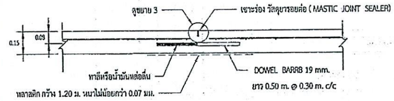
ขยายรอยต่อ CONTRACTION JOINT
