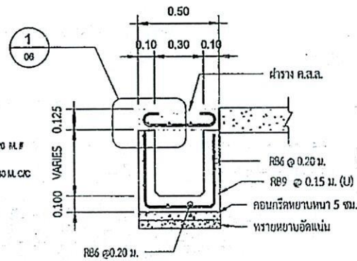
ขยายร่างระบายน้ำ 1:20
