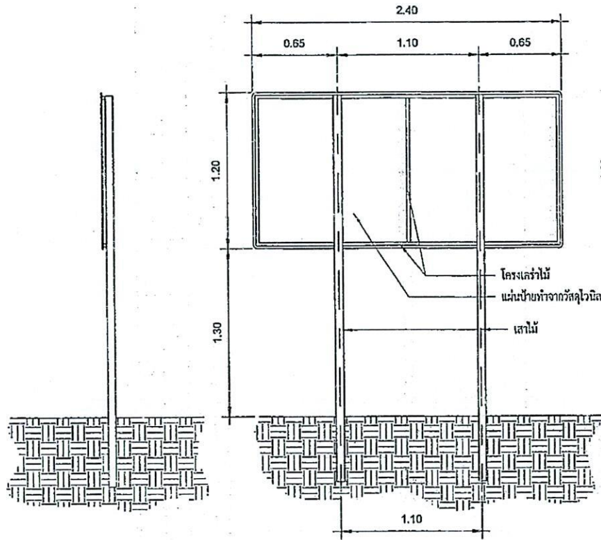
รูปด้านข้าง 1:25
