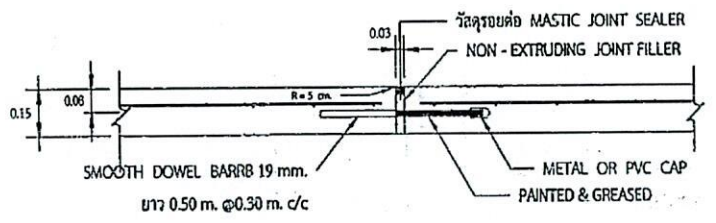
ขยายรอยต่อ EXPANSION JOINT
