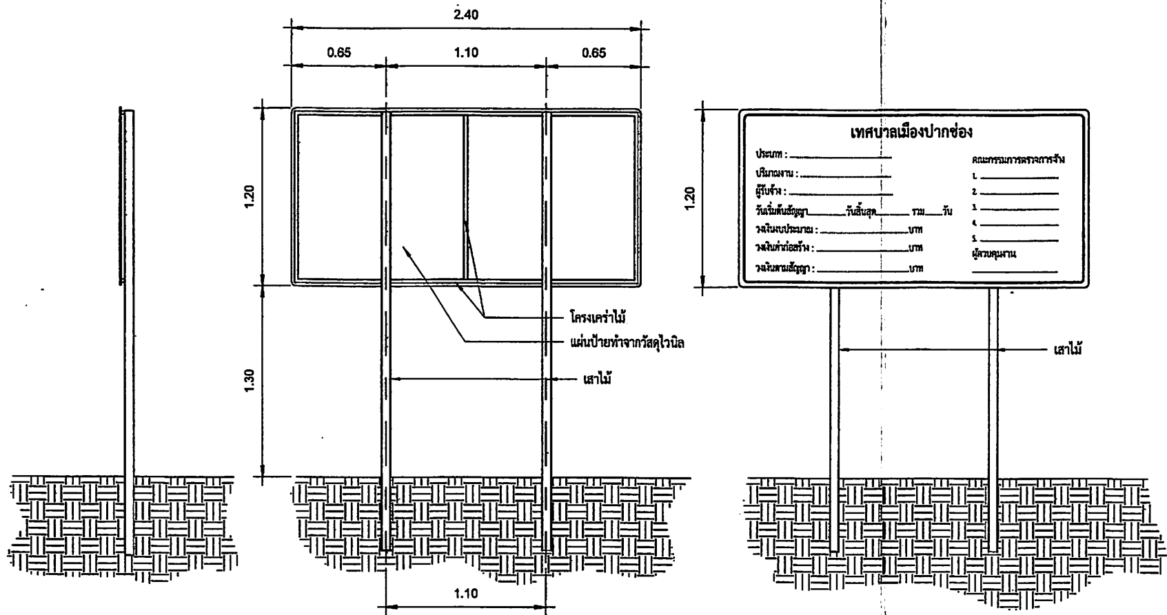
รูปด้านข้าง 1:25
