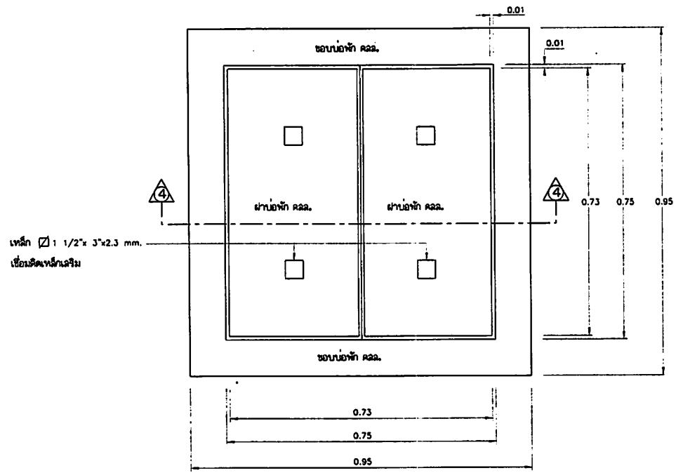
ขยายฝาบ่อพัก 1:10
