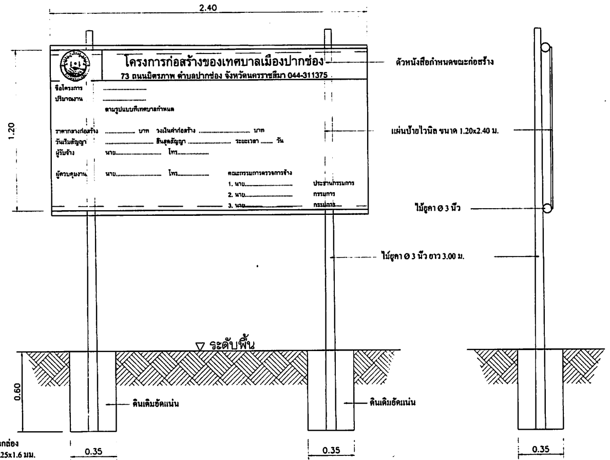
ป้ายประชาสัมพันธ์โครงการ มาตราส่วน 1:20
