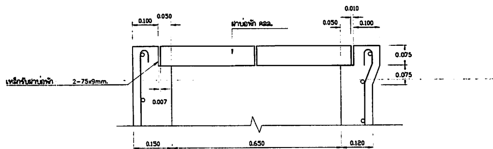
ขยายรูปตัดฝาบ่อพัก 1:10
