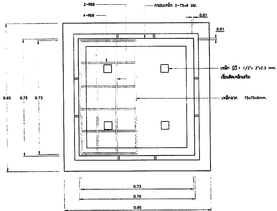
ขยายฝาบ่อพัก 1:10
