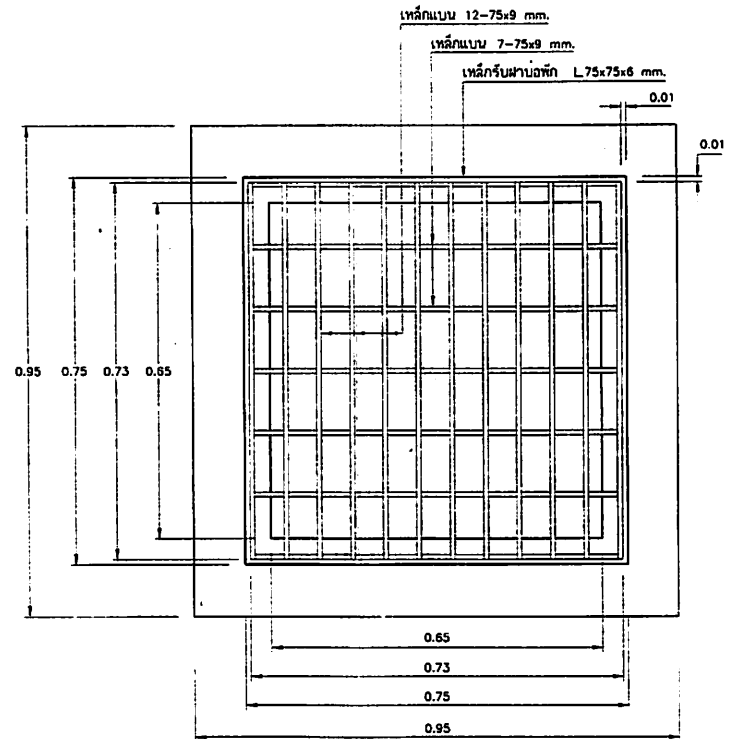
ขยายผ้าบ่อพัก 1:10
