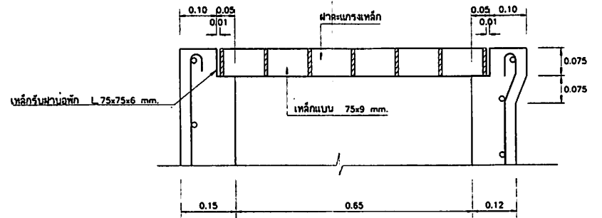
ขยายรูปตัดผ้าบ่อพัก 1:10
