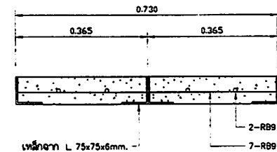
ขยายฝาบ่อพัก 1:10
