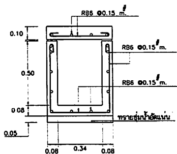
แบบขยายบ่อพักเล็ก 1:25
