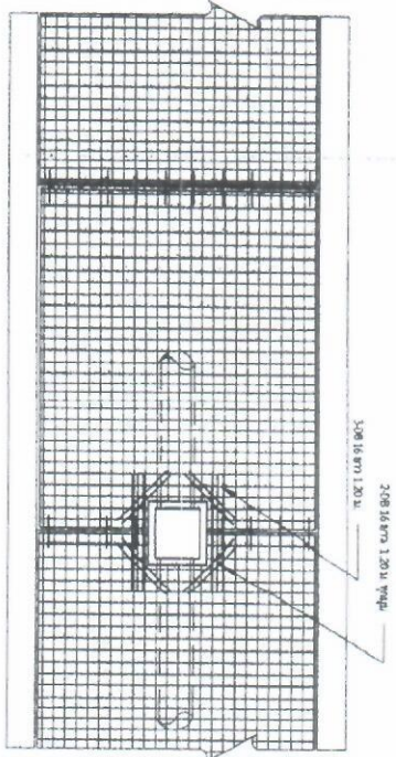
แบบขยายปากข้อพัก กรณีข้อพักอยู่ระหว่างรอยต่อแผ่นคอนกรีต
