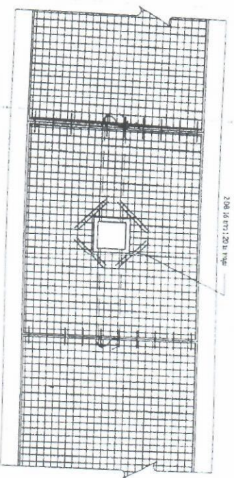
แบบขยายปากบ่อพัก กรณีบ่อพักอยู่กลางแผ่นคอนกรีต
