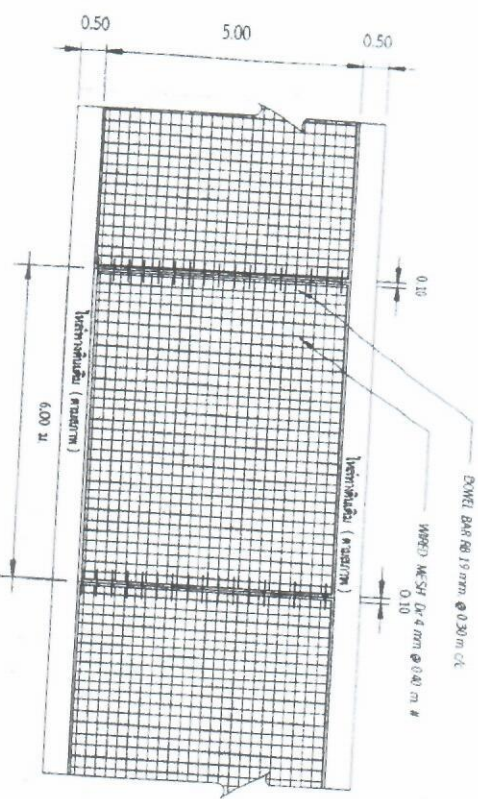
แบบขยายการเสริมเหล็กบนคอนกรีต
