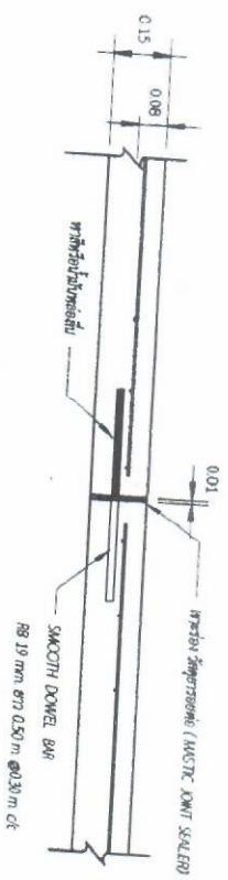
ขยายรอยต่อ CONSTRUCTION และ JOINT CONTRACTION JOINT
